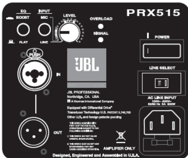
Panel wejściowy PRX515
