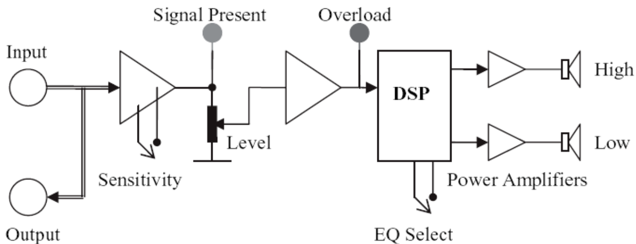
Schemat blokowy
